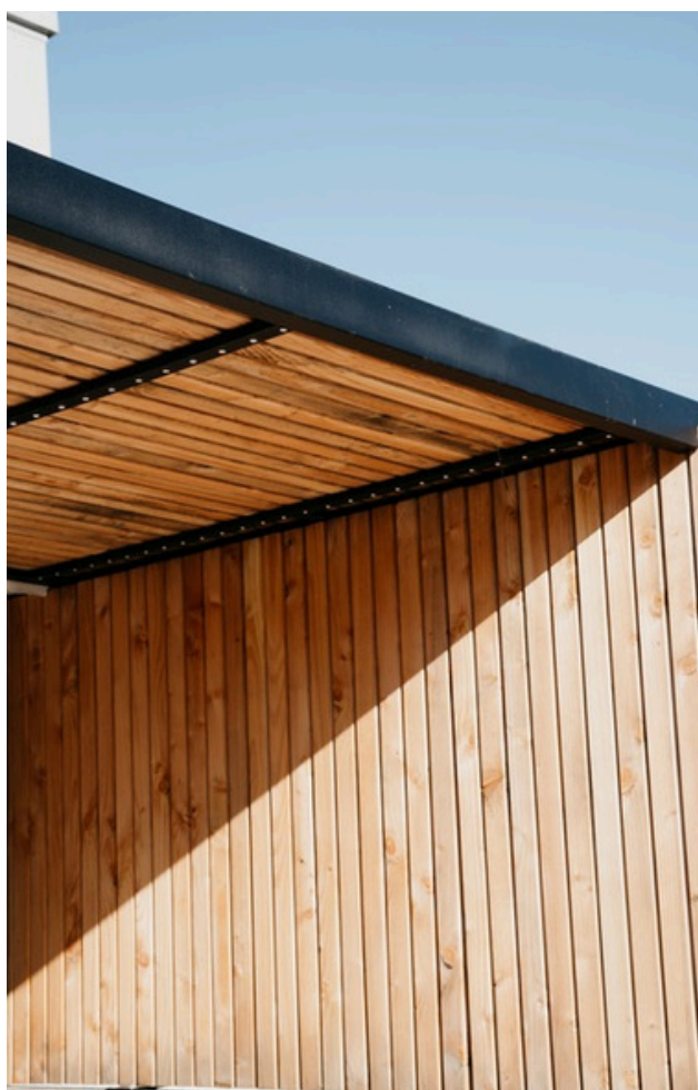
Pergola structure en acier thermolaqué + Liteaux douglas biaisés
