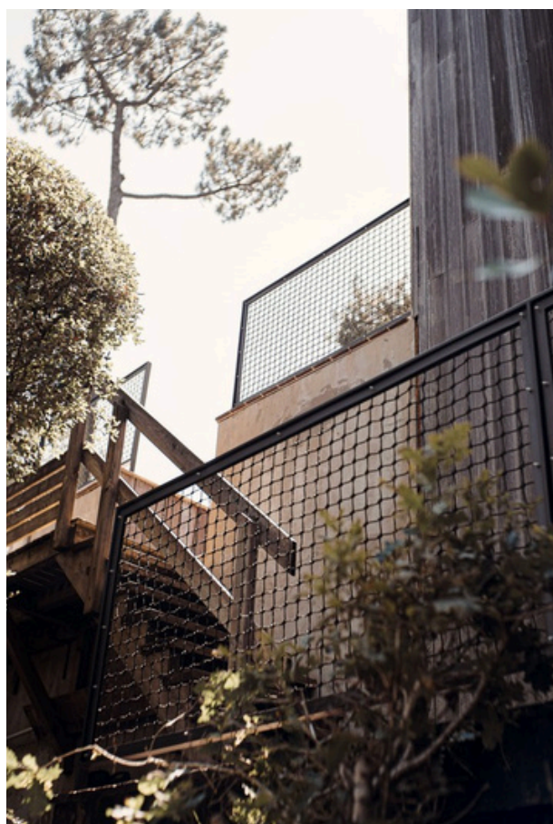
Garde-corps en filet + thermolaquage RAL 1019
