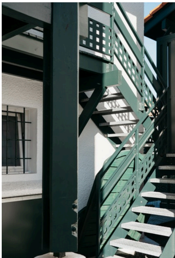
Garde corps en tôle perforée + thermolaquage RAL 6012
